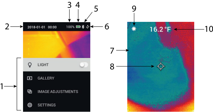
Рисунок 4.2 Дисплеи TG275
